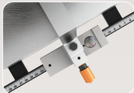
Squadro con riga millimetrata e lente di ingrandimento Guide avec échelle graduée et lentille Fence with graduated scale and lens Anschlag mit Millimeterlinie und Lupe Guía con escala graduada y lente
