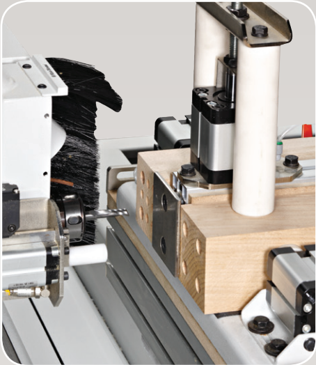
Forature e fresature di testa
